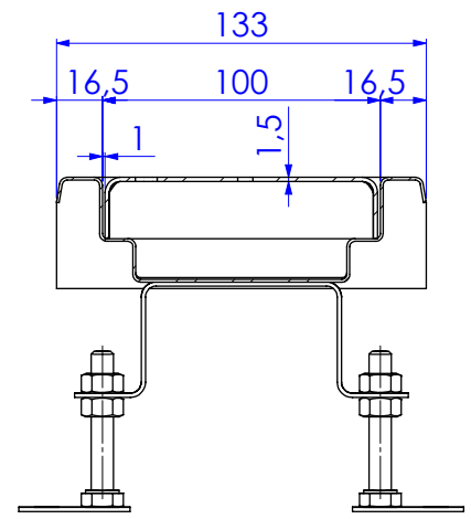
ŘEZ B-B
